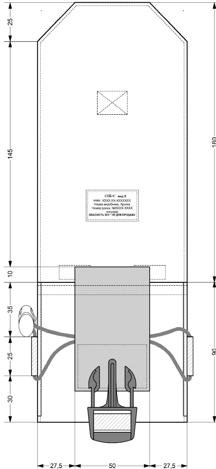
Рисунок Д2.1 – Вид спереду
