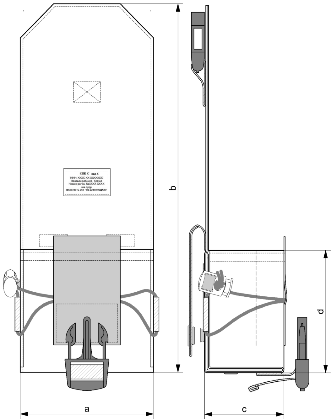
Рисунок Д1.2 – Габаритні розміри
