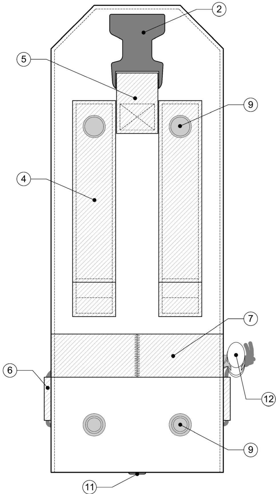
Рисунок Д3.3 – Позначення деталей предмета
