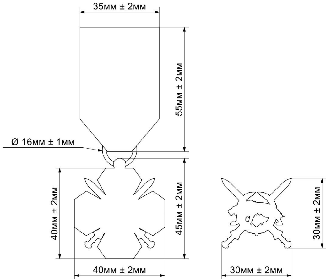
Рисунок Д1.3 – Лінійні розміри предмета
