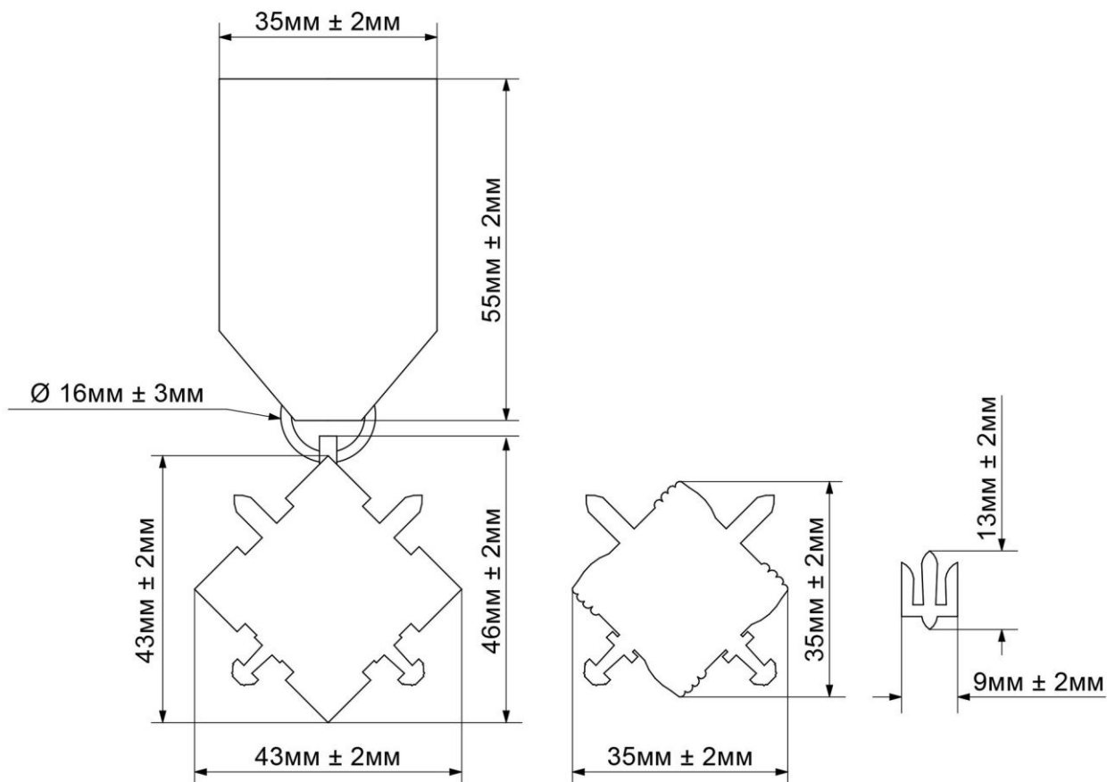
Рисунок Д1.2 – лінійні розміри предмета
