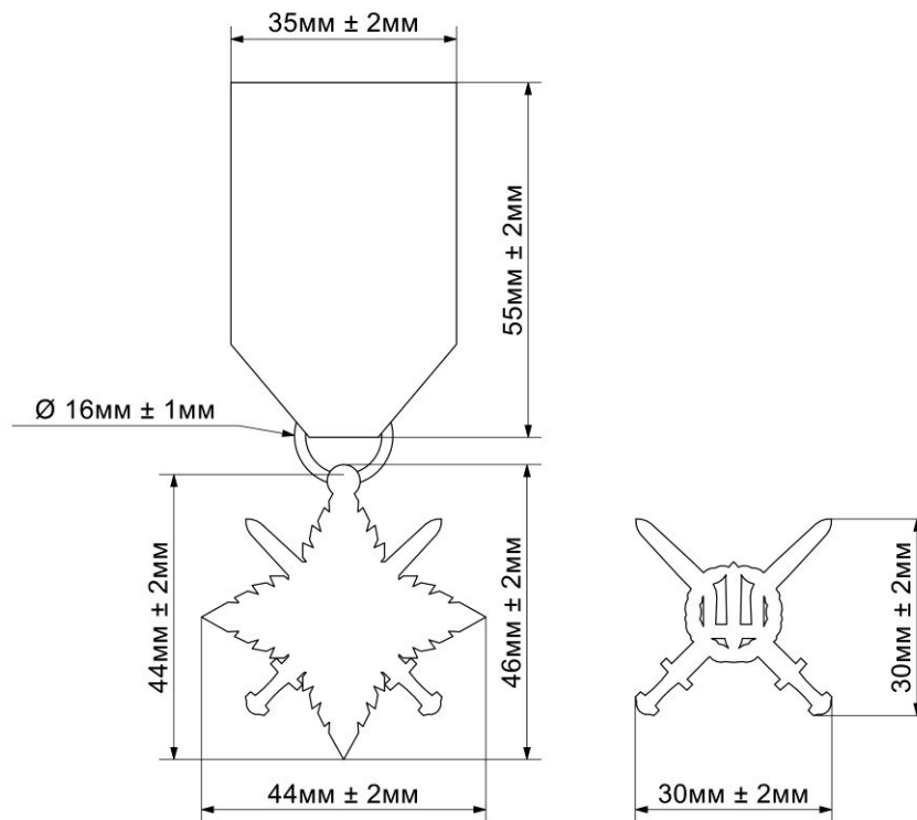
Рисунок Д1.3 – Лінійні розміри предмета
